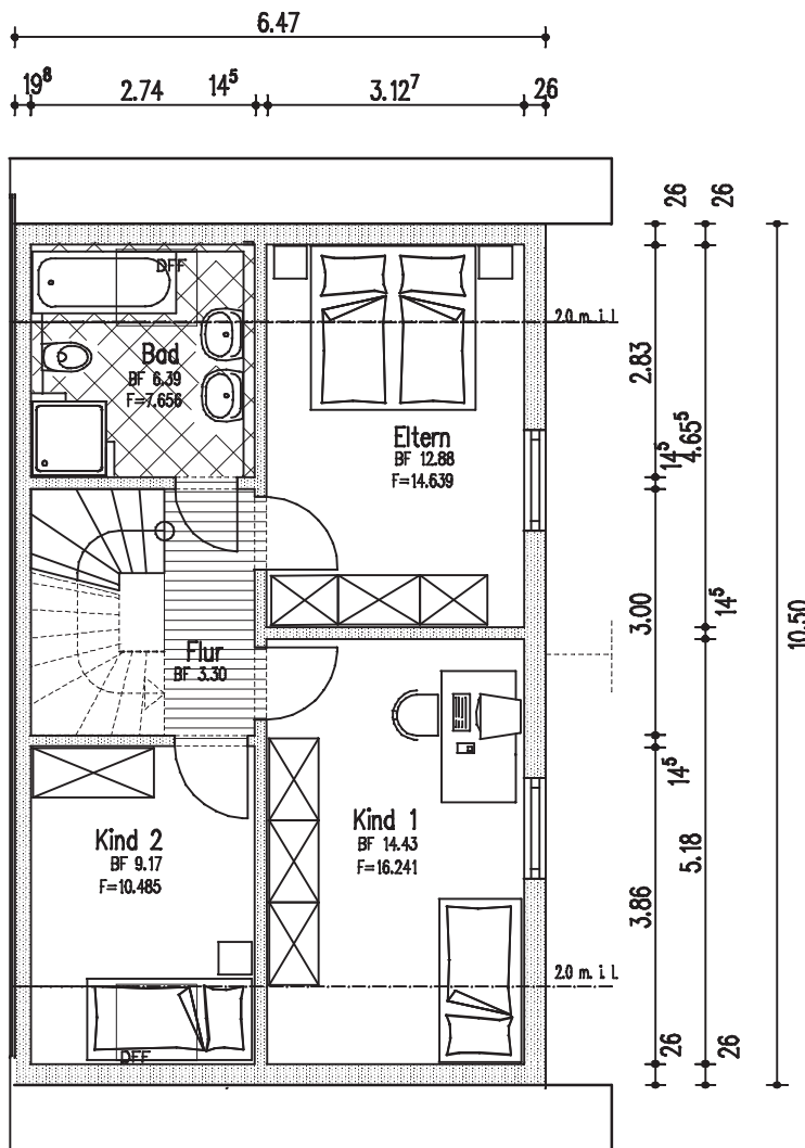
Obergeschoss
